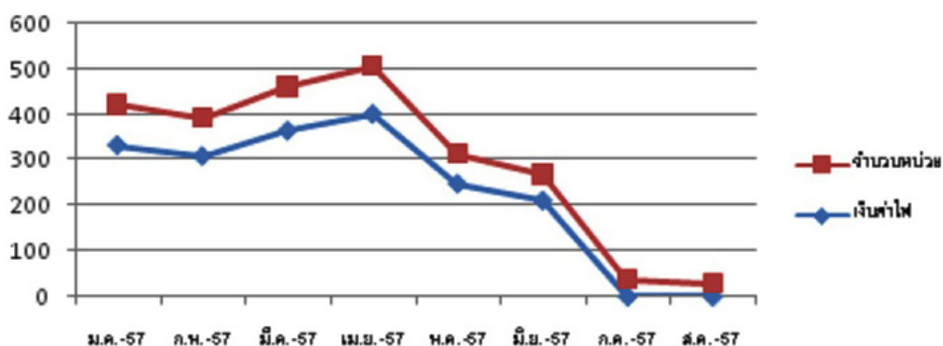
กราฟที่ 1 การเปลี่ยนแปลงค่าไฟฟ้าครัวเรือนของอาสาสมัครปฏิบัติทดลองที่ติดตั้งโซล่าเซลล์เมื่อเดือนเมษายน 2557
